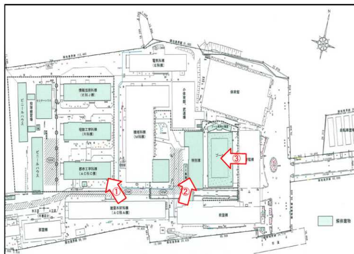
現校舎配置図
