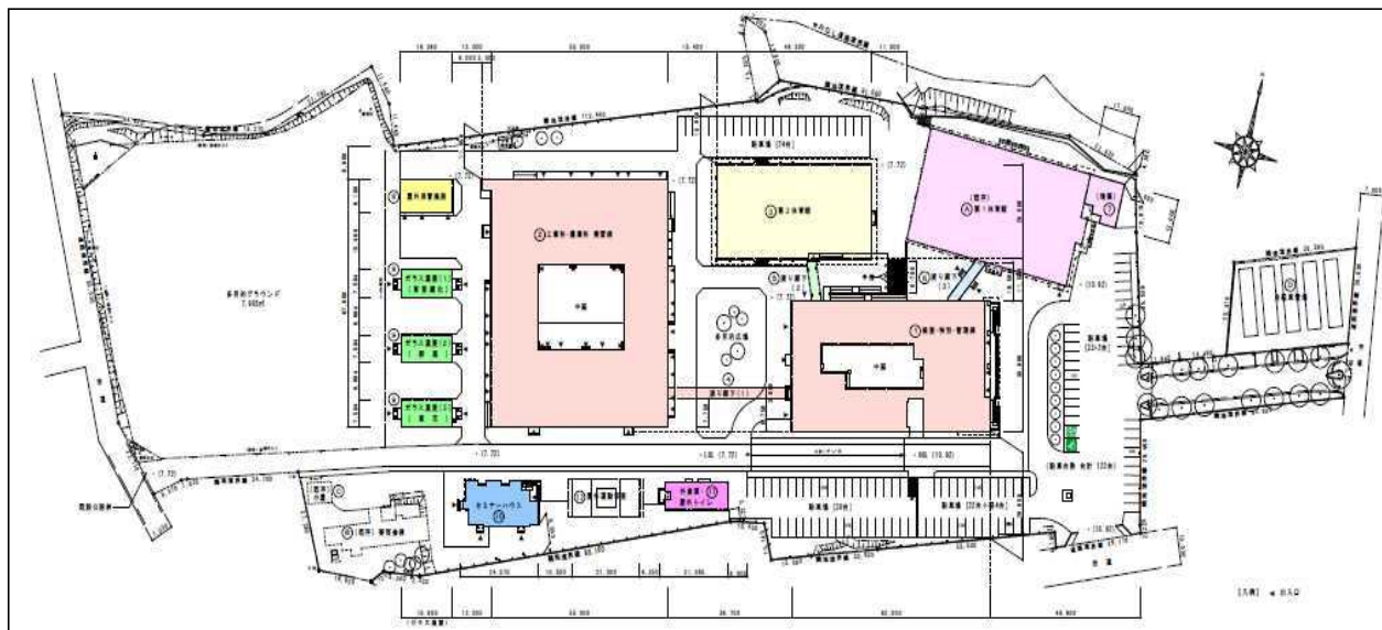
統合校配置計画図
